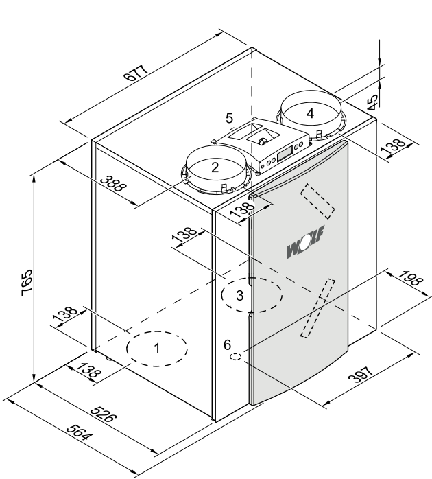
CWL-300/400 Excellent Rechtsausführung 2/2
