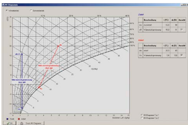
HX-Diagramm
