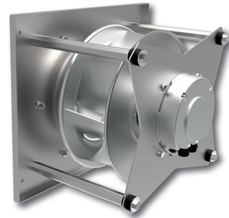
Freilaufendes Rad des Typs GKHM mit energieeffizientem EC-Motor
